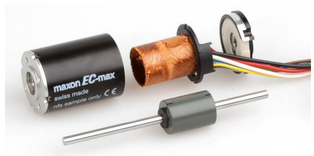
Bottom right: maxon EC-max 30 motor
